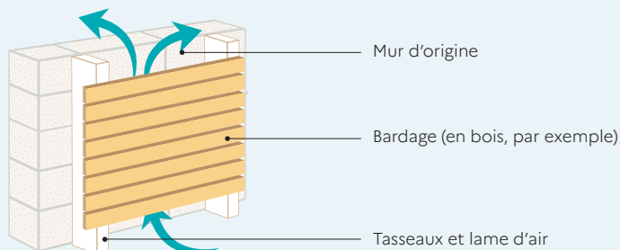
Isolation avec bardage léger sur une façade
